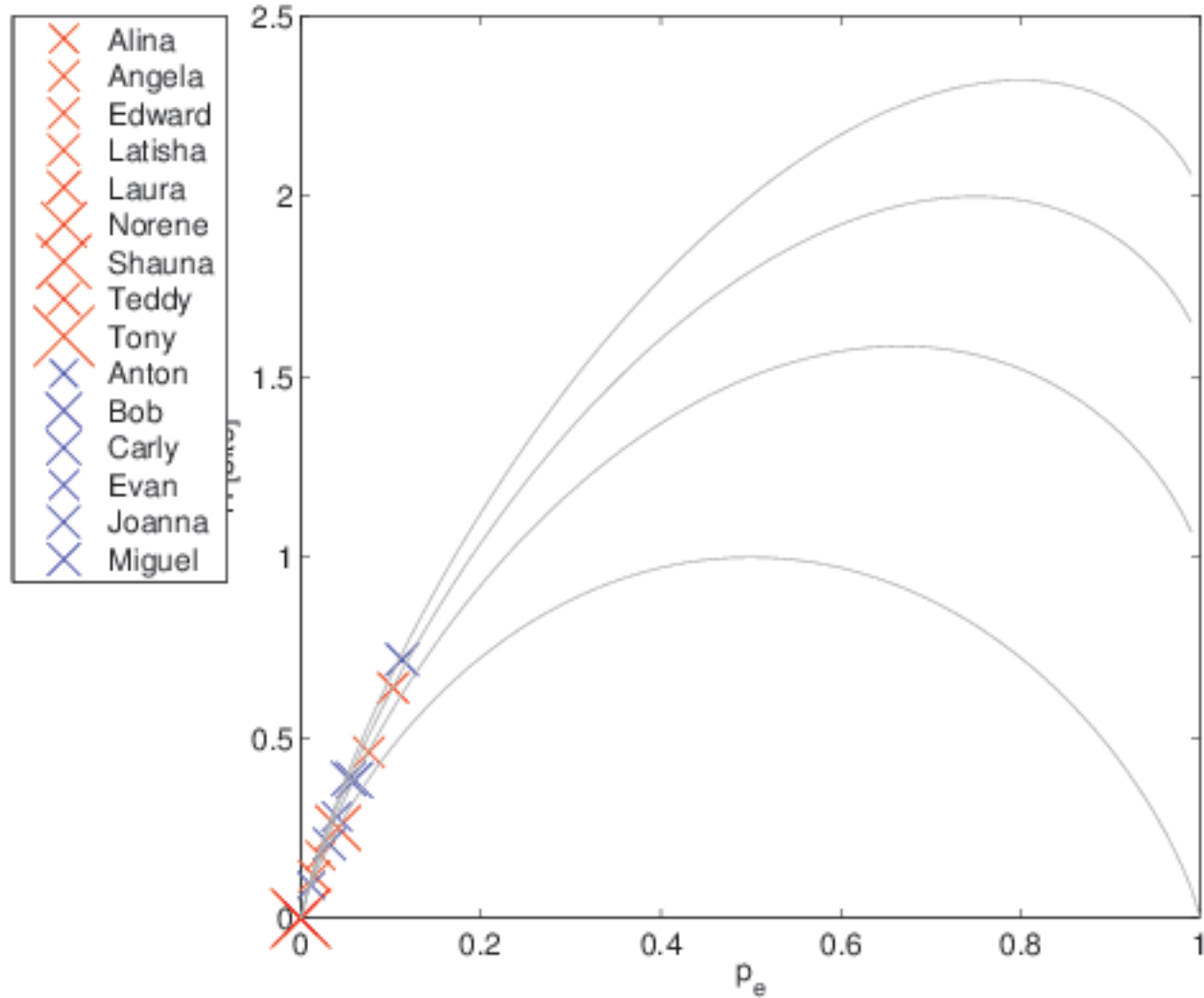
H(p_e) for Letter (d) in Initial Position
