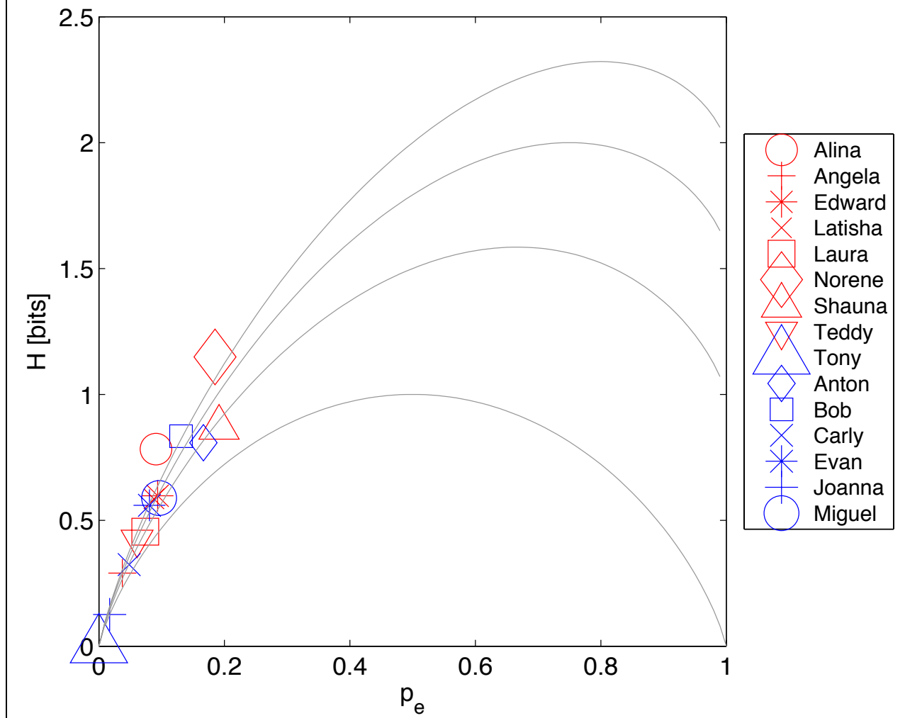
H(p_e) for Letter (d) in Final Position
