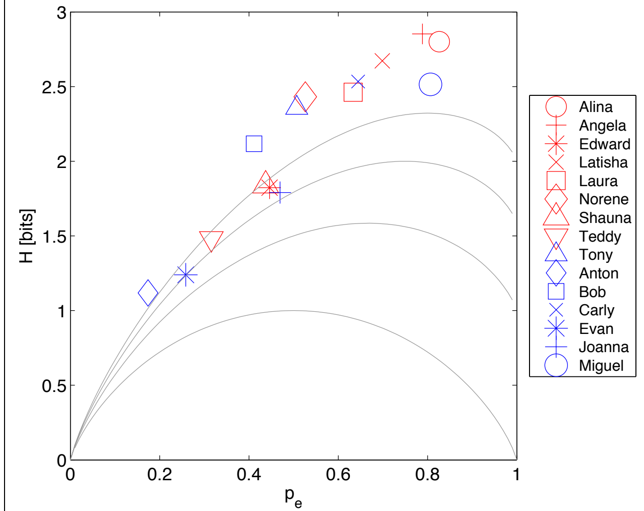
H( p_e ) for Letter (D) in Final Position
