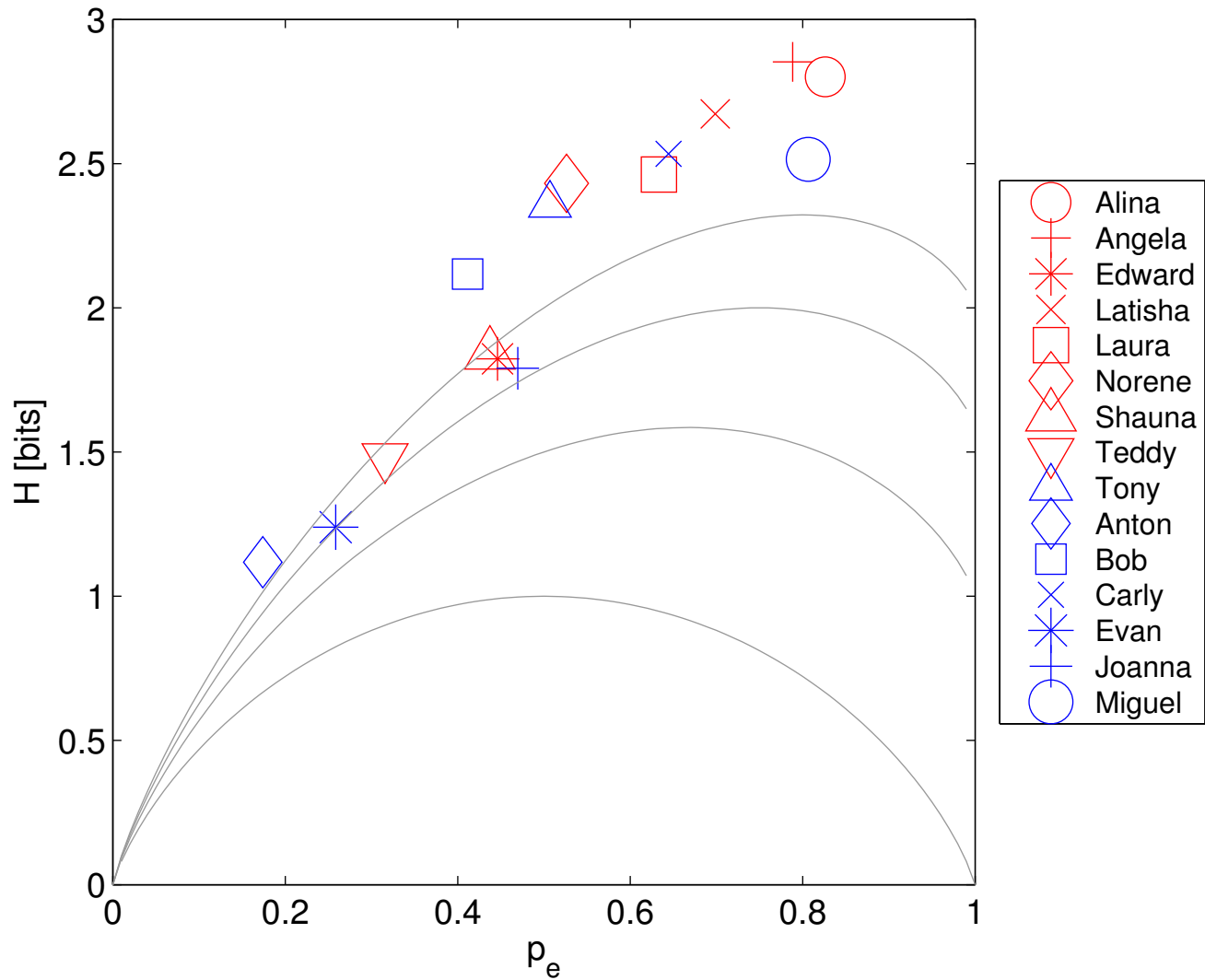
H(p_e) for Letter (D) in Final Position
